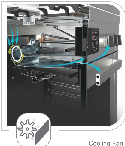
Cooling Fan
